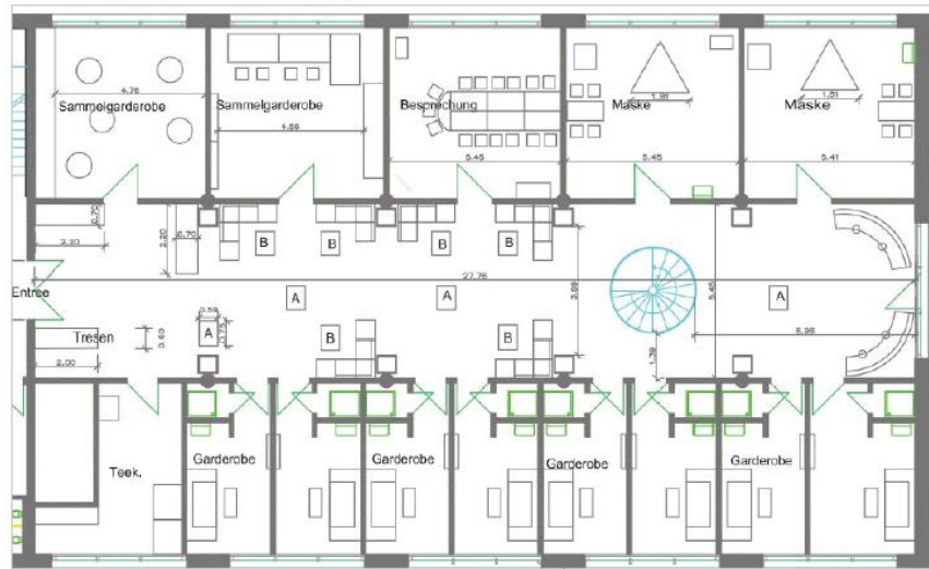
1. Obergeschoss: VIP-Bereich
